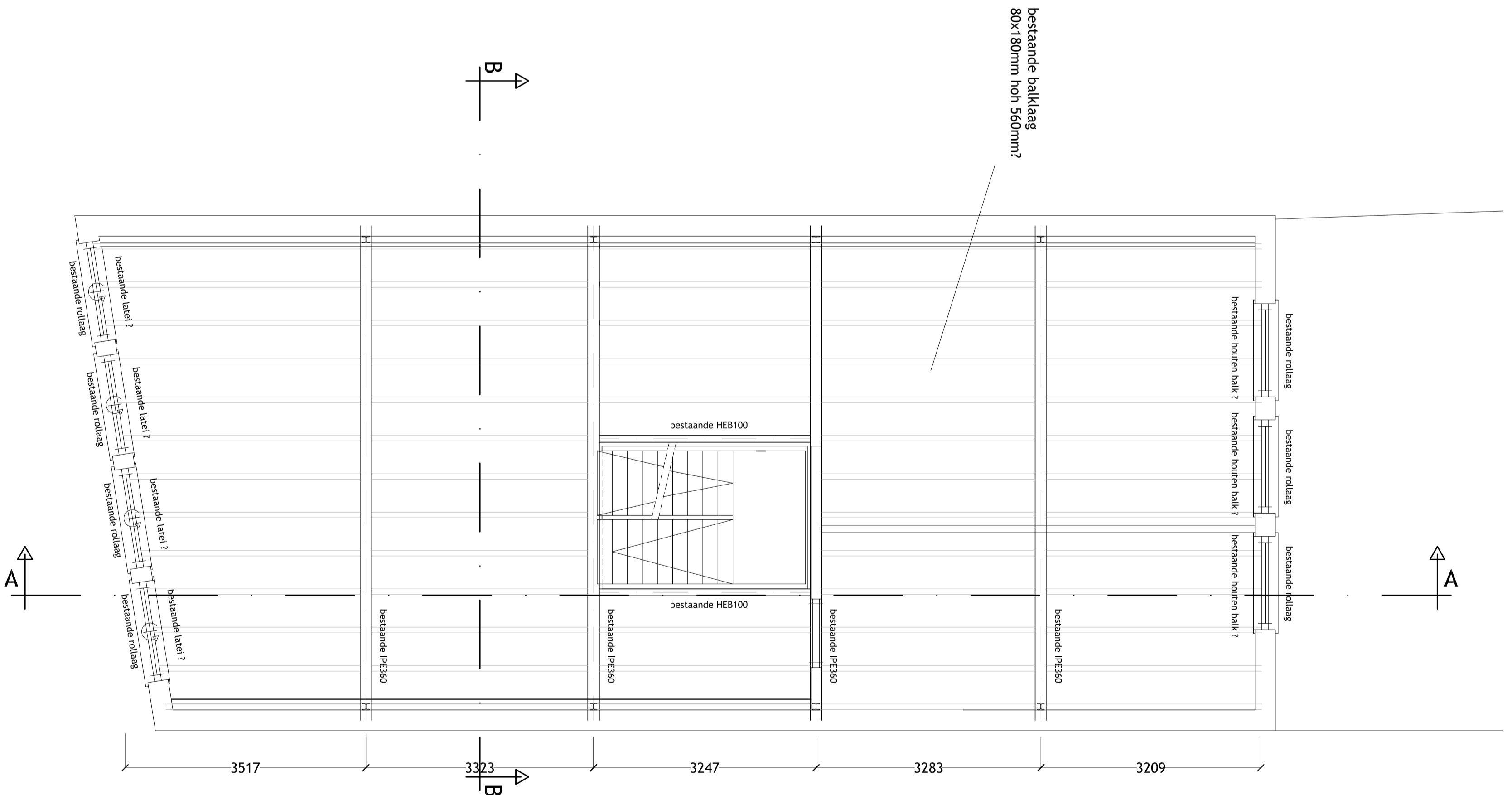
tweede verdieplingsvloer
