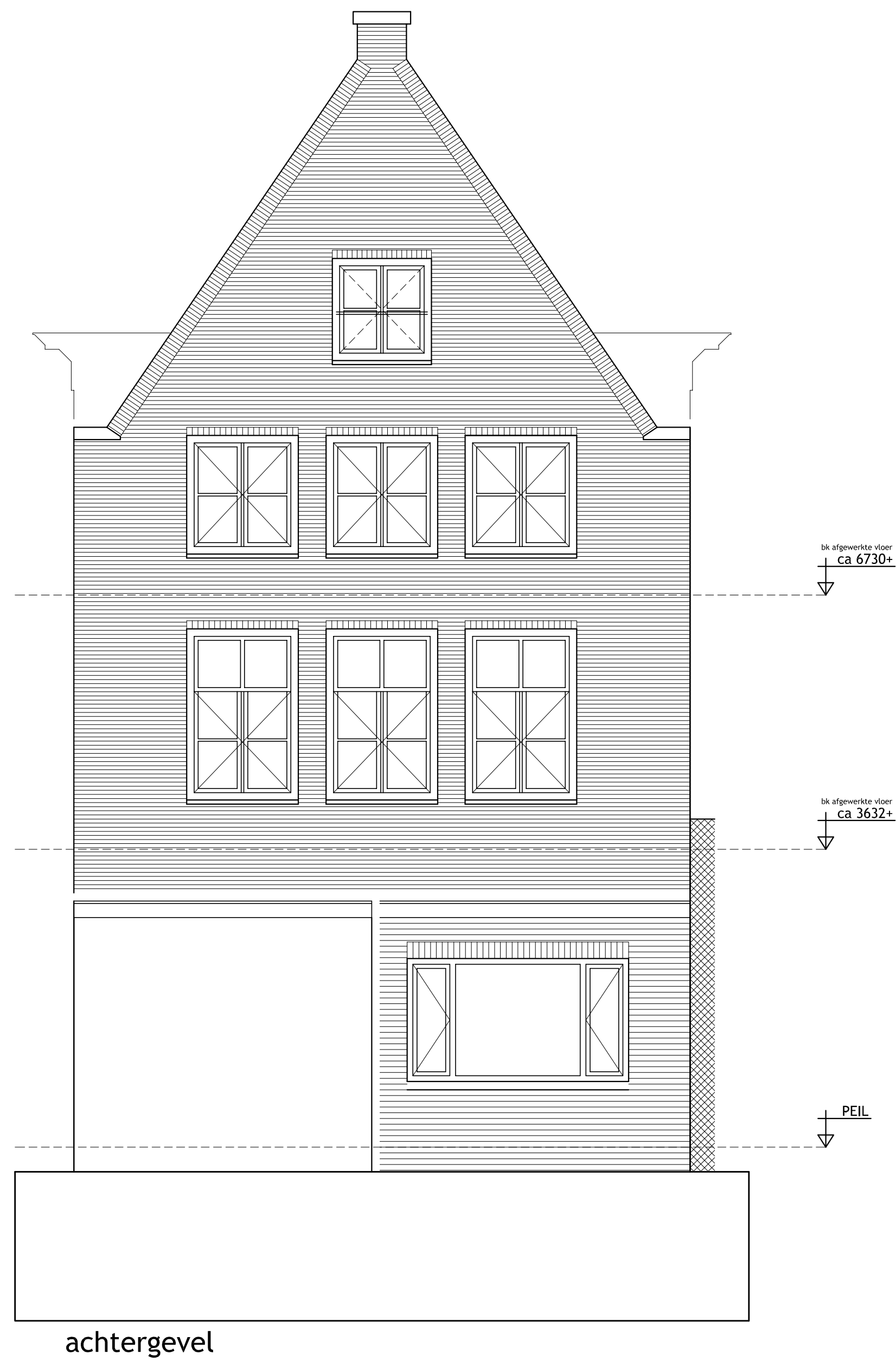
achtergevel
