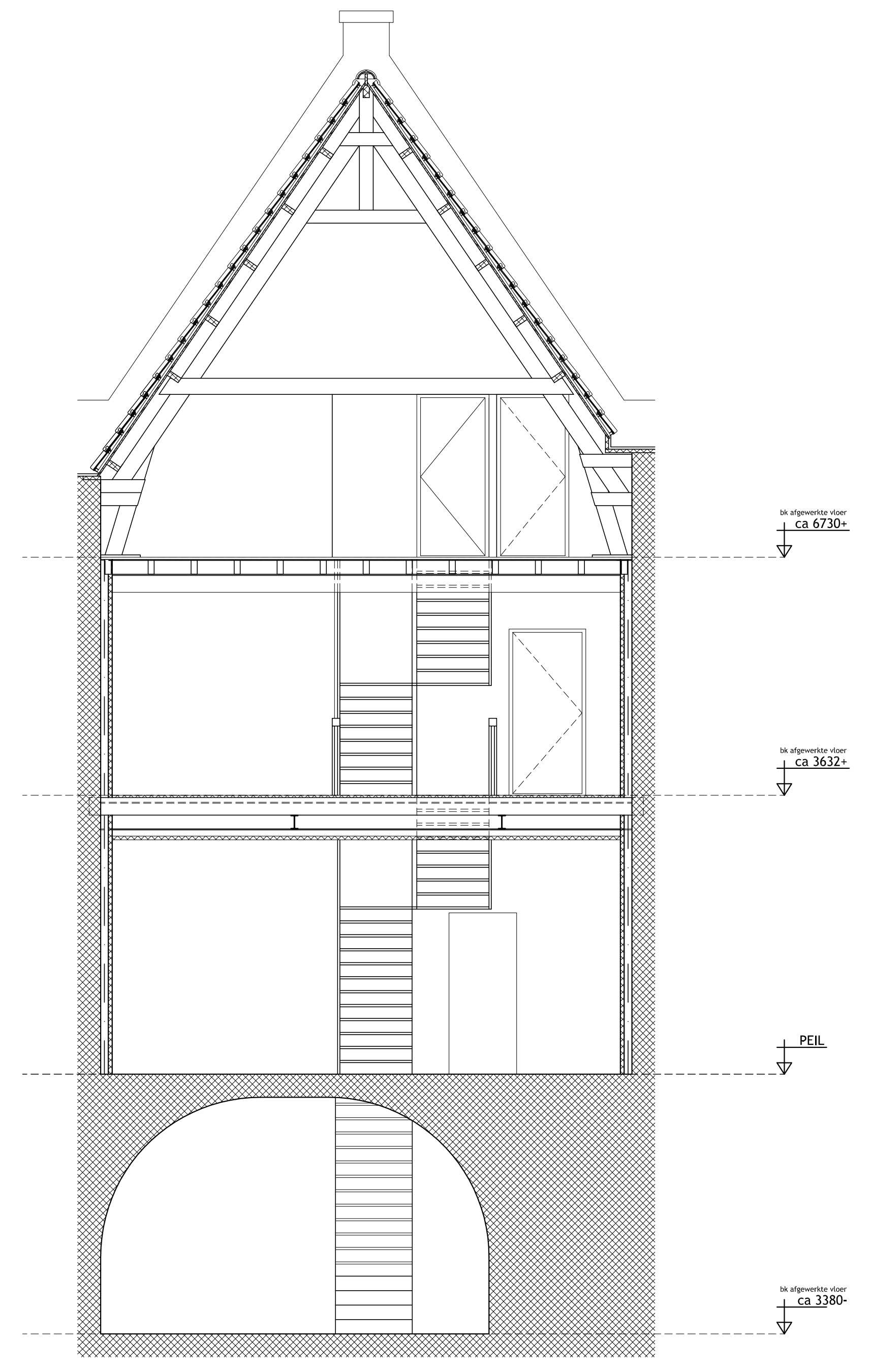
doorsnede B-B
